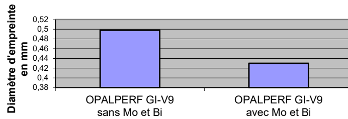
Usure selon test 4 billes (ASTM D 4172)
